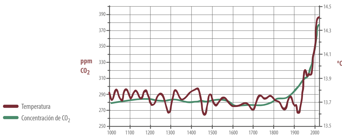
Figura 3. Temperatura media global y concentración de CO 2 del año 1000 al 2000
