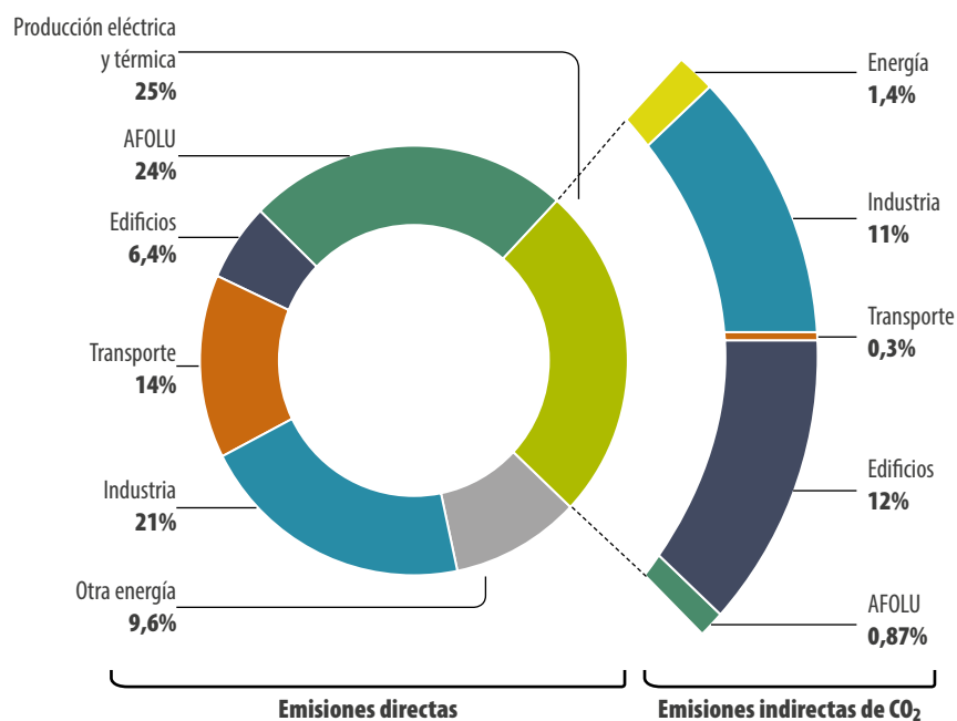
Figura 7. Emisiones de gases de efecto invernadero por sectores económicos
