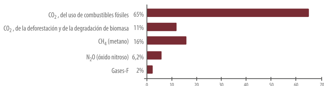
Figura 2. Parte proporcional que representan diferentes GEI antropogénicos
